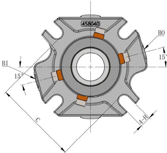
K向/View K 比例不符/NO SCALE
