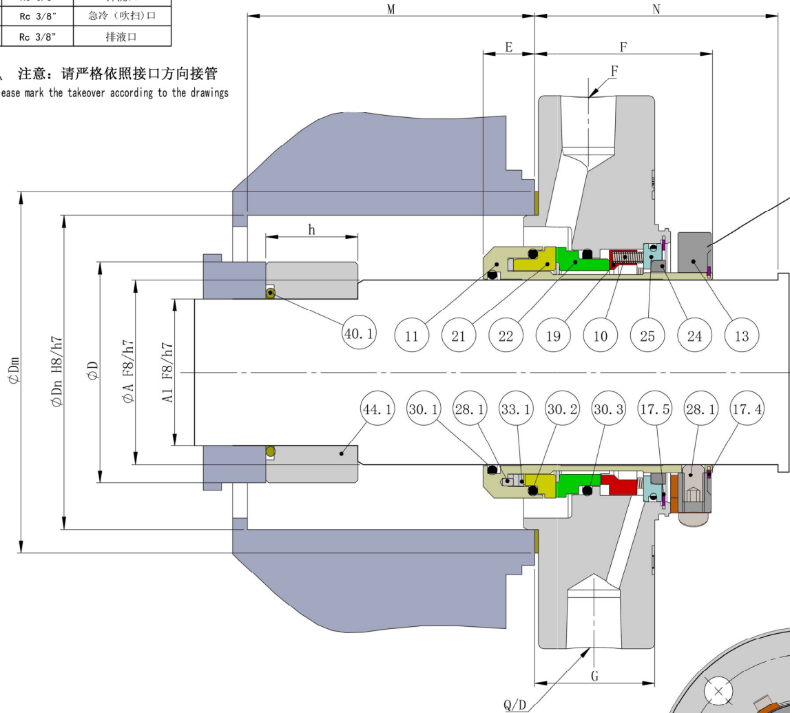
剖面 A-A
